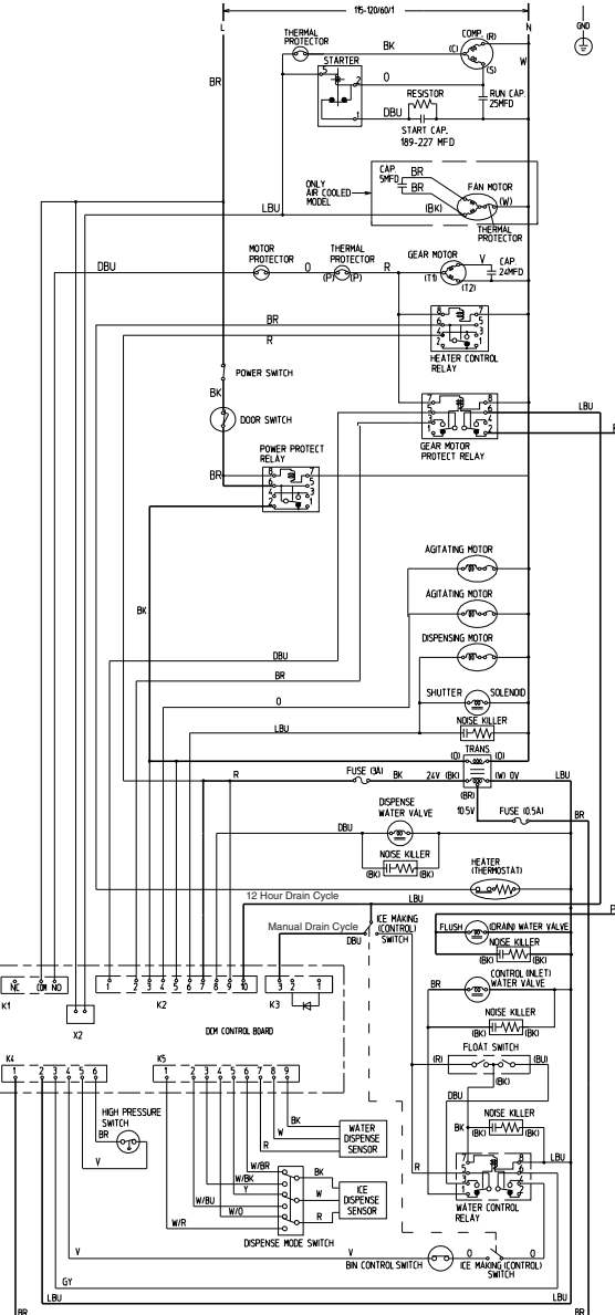
DCM-750BAH-OS, DCM-750BWH-OS
